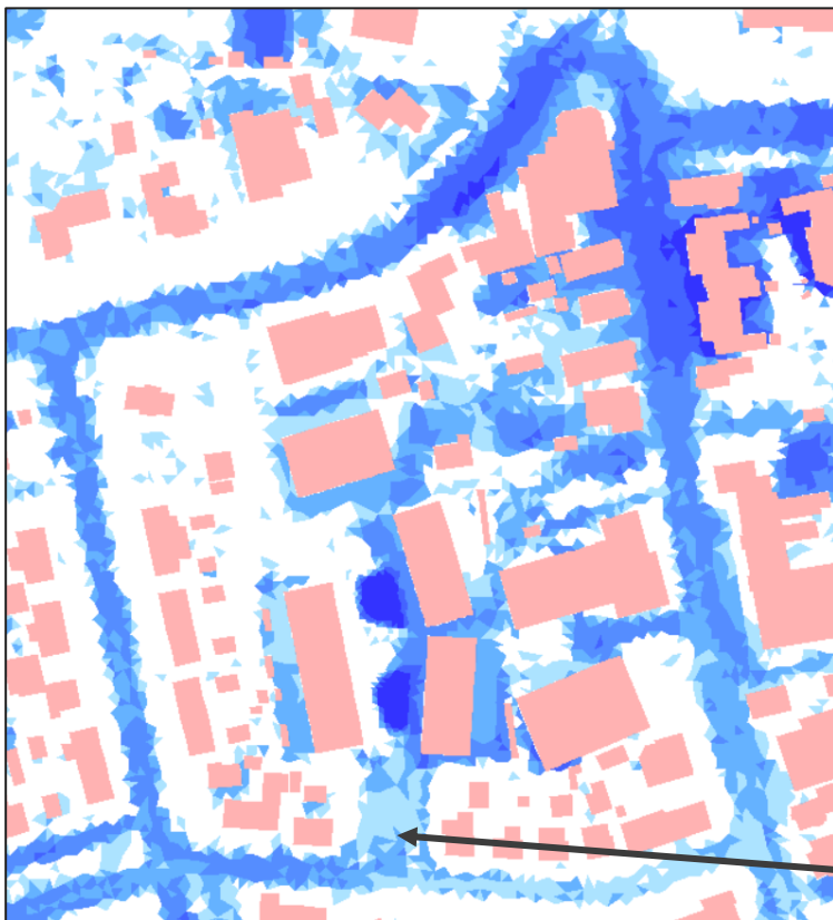
Afbeelding 3.6: Resultaat stresstest 90 mm in 1 uur, eerste ontwerp
